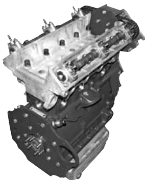
Fig.: AT-Motor / Exch. Engine MGA Twin Cam
