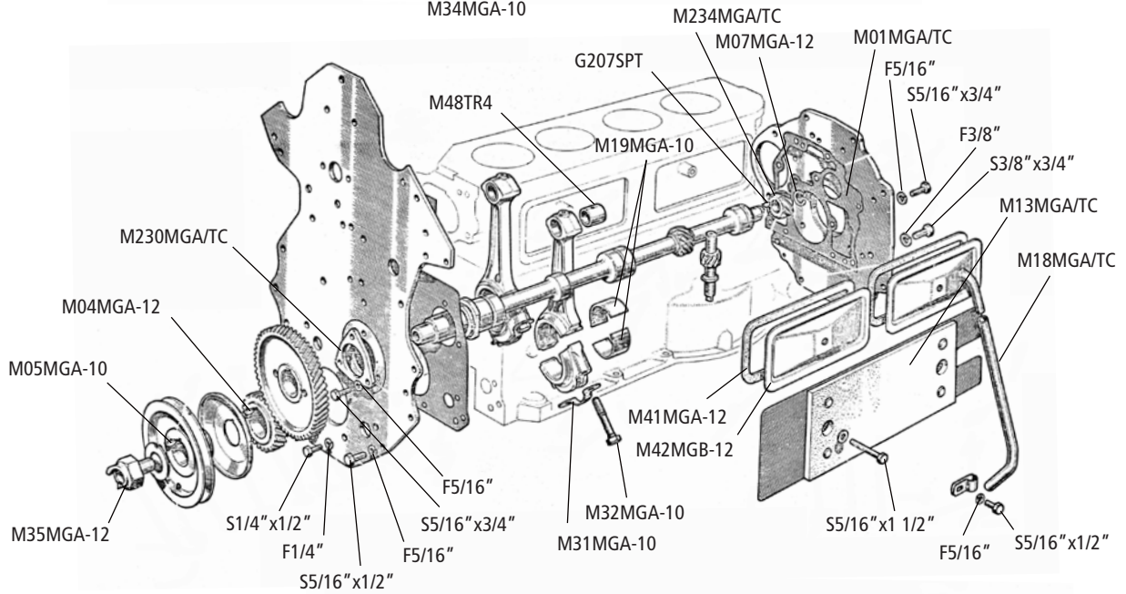
Fig.: AT-Motor / Exch. Engine MGA Twin Cam
