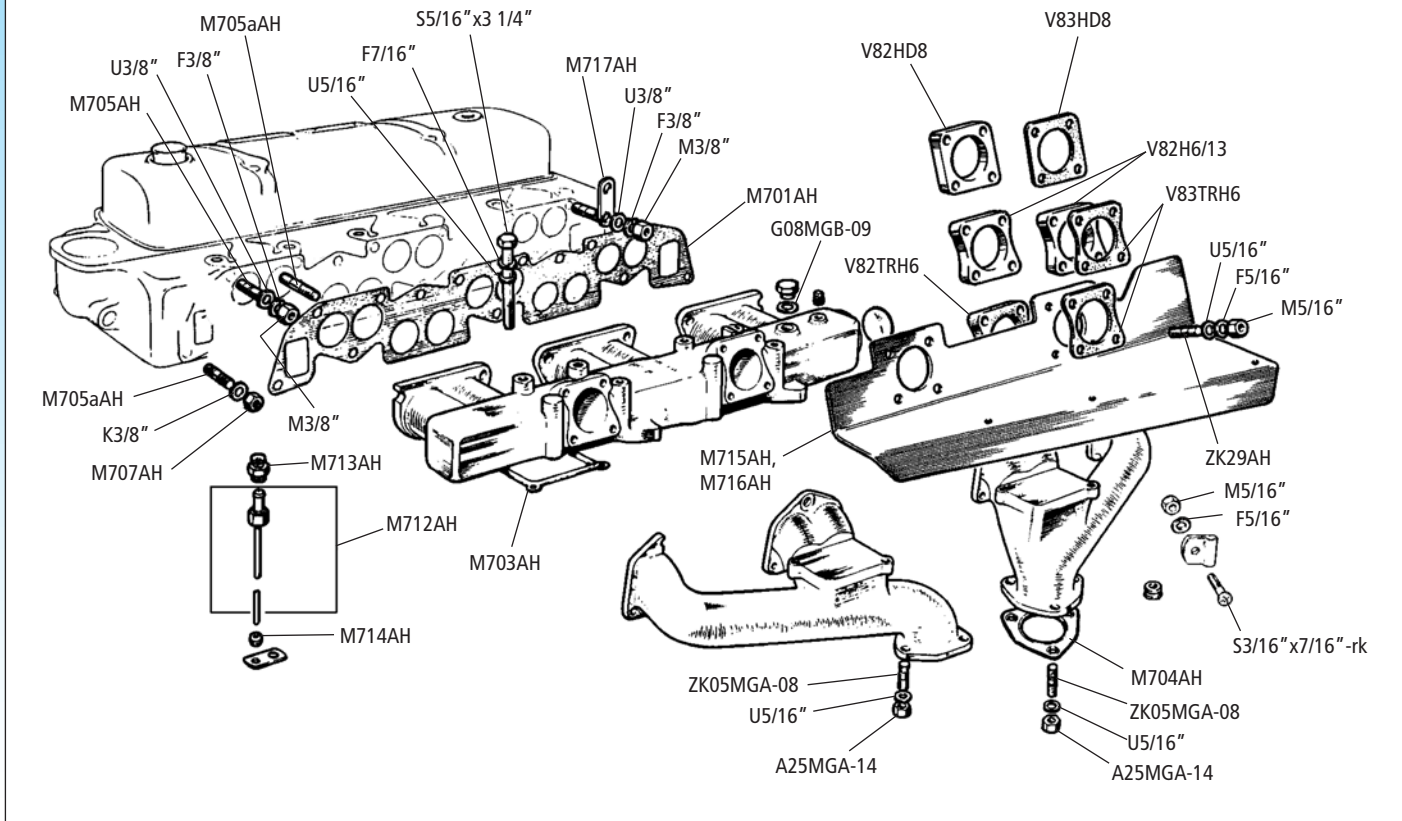
Ansaugbrücke, Auspuffkrümmer / Manifolds BN4&gt;48863, BN6, BN7, BT7, BJ7, BJ8
