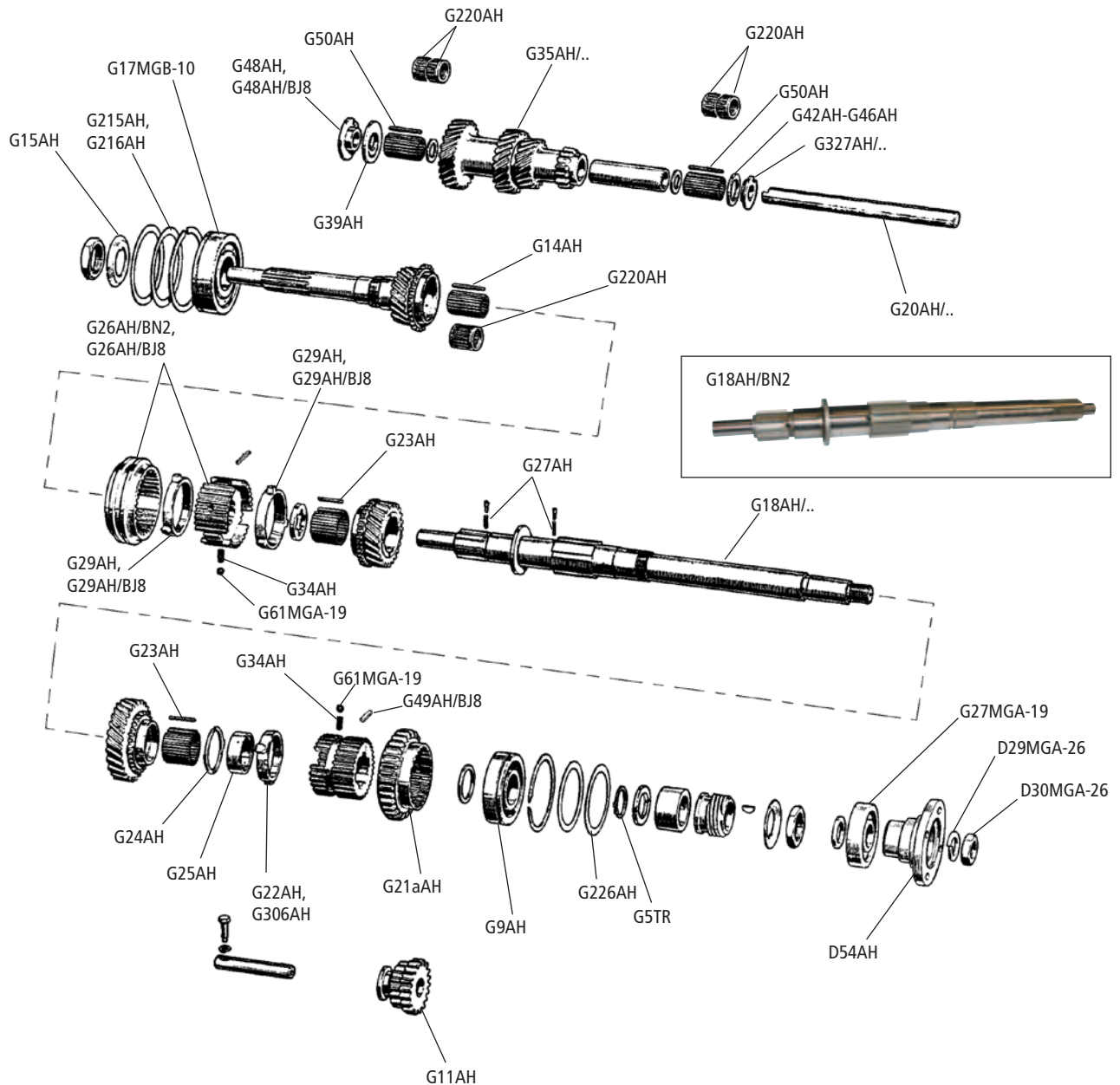
Getriebe 4-Gang / Internal Gearbox 4 speed BN2, BN4, BN6, BN7, BT7, BJ7, BJ8
